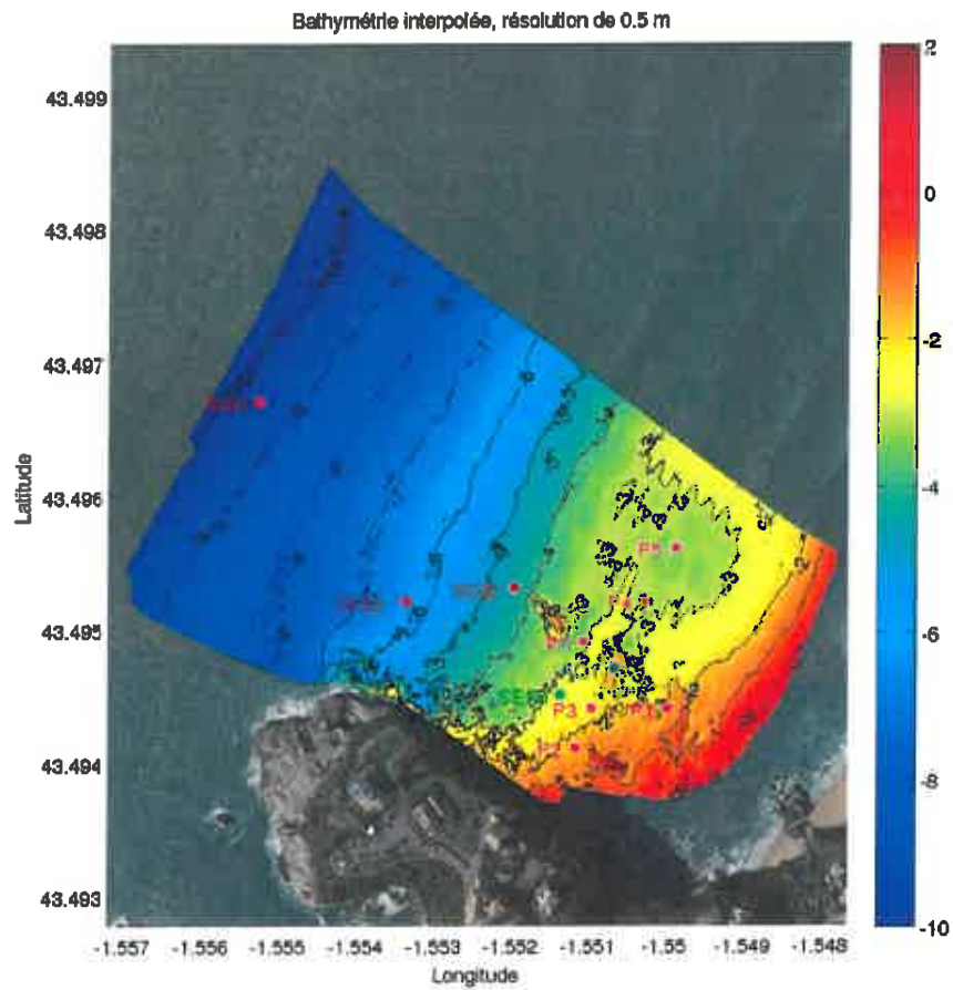
Bathymétrie du site d'étude et disposition des capteurs. 6 capteurs de pression (P) et 5 courantomètres (SIG, SEN, AQ)
