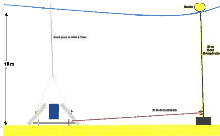
Schéma représentant le mouillage d'un instrument
